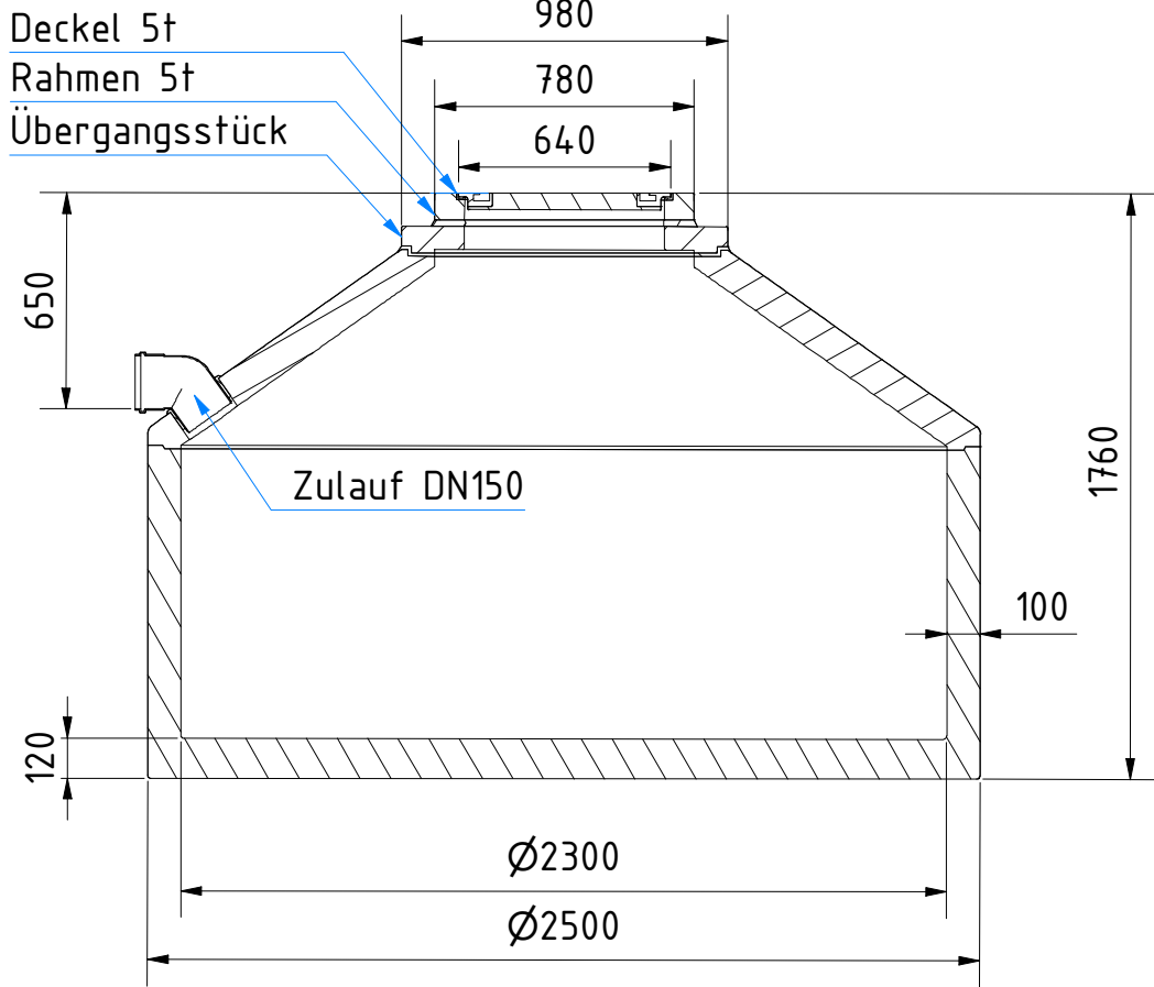
H-H ( 1 : 25 )
